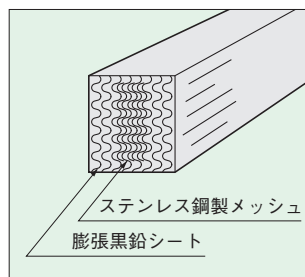
図1 TOMBO No. 2205の断面図
