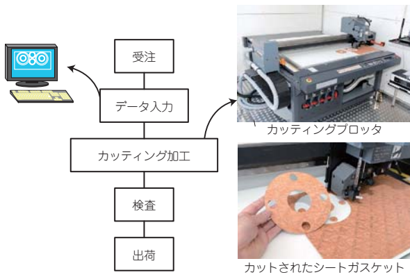
図2 「GASKET工房™」の加工フロー図
